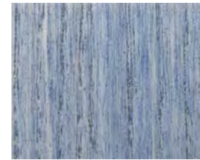
Céanothe
